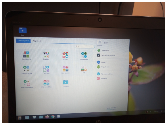
Kuva 5: Ohjelmistot
