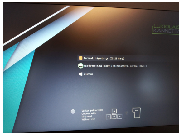
Kuva 1: Käynnistysvalikko
