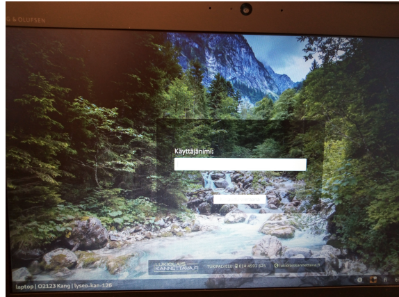
Kuva 2: Kirjautumisikkuna
